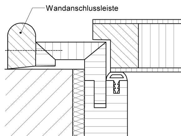
Bild 3 Zargenanschluss mit Zierleiste
