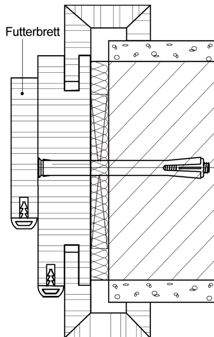
Bild 8 Türzarge mit zusätzlicher mechanischer Befestigung
