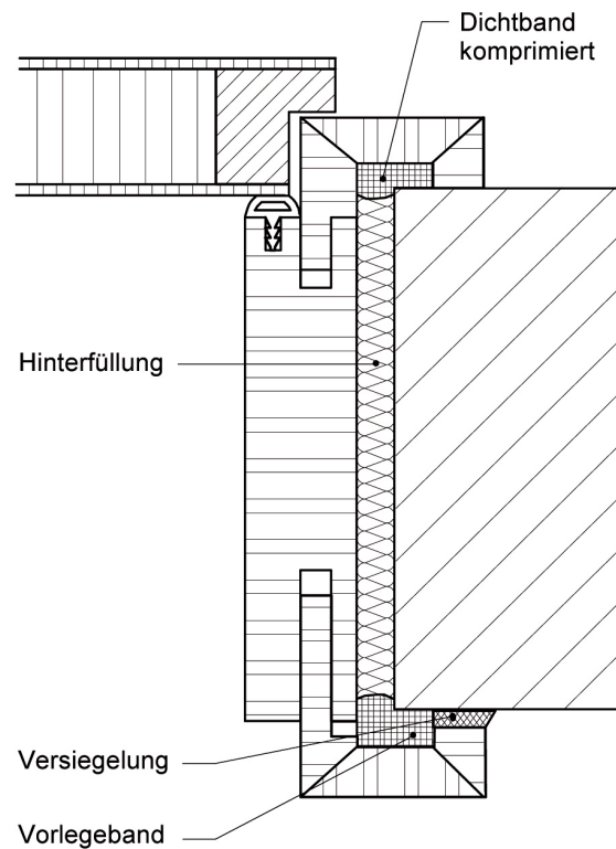
Bild 9 Abdichtungsmaßnahmen zwischen Zarge und Mauerwerk bei einer Schallschutztür
