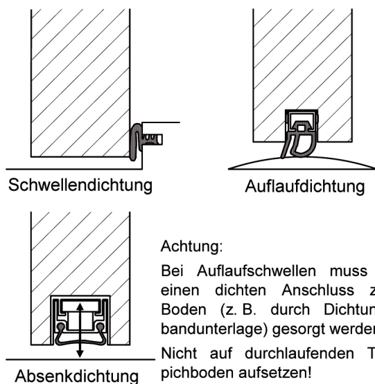
Bild 10 Abdichtungsmöglichkeiten zwischen Tür und Fußboden
